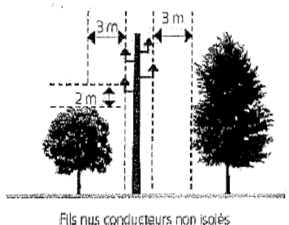
Fils nus conducteurs non isolés
